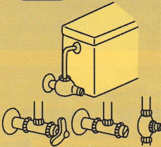
止水栓の種類
